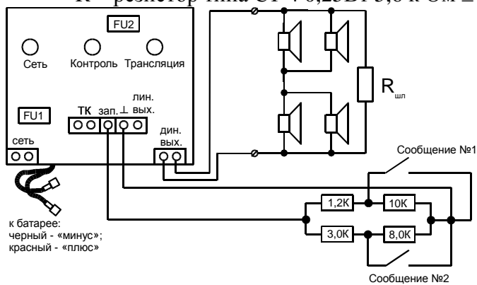
Схема внешних соединений прибора «СОНАТА-К-Л», рис.1
