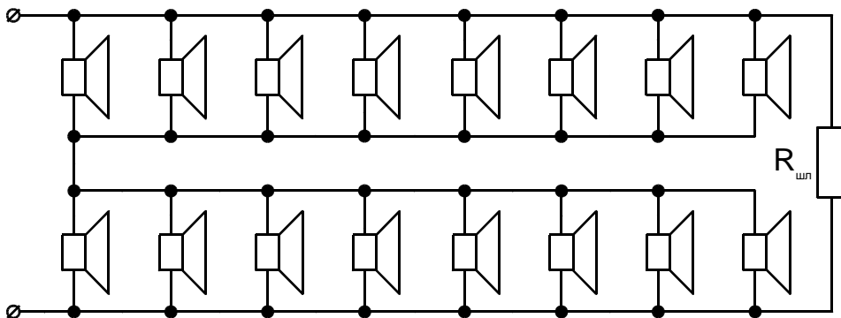
Подключение шестнадцати акустических оповещателей Z_H=8\text{ Ом} , P_H=3\text{Вт} ; P_{\text{вых}} \approx 1,5\text{ Вт/оповещатель} – рис.6
