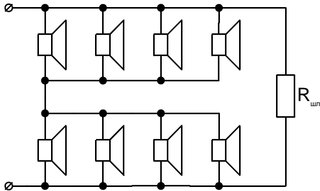
Подключение восьми акустических оповещателей Z_H=4\text{ Ом} , P_H=3\text{Вт} ; P_{\text{вых}} \approx 3\text{Вт/оповещатель} – рис.5
