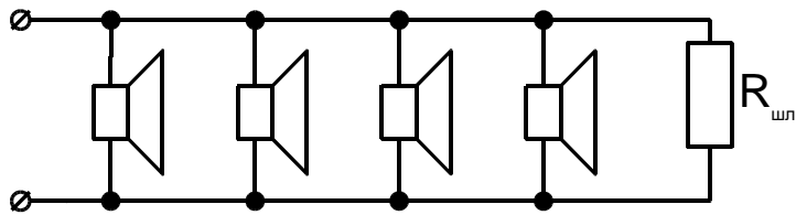
Подключение четырех акустических оповещателей Z_H=8\text{ Ом} , P_H=8\dots 10\text{Вт} ;
