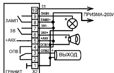
Рис.3 Подключение лампы, Призмы-200И, сирены, табло с питанием 12В.
