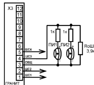
Рис.6 Подключение токопотребляющих пожарных извещателей
