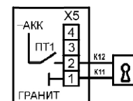
Рис.4 Подключение пассивных электромагнитного замка
