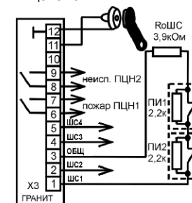
Рис.5 Подключение пассивных пожарных извещателей
