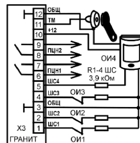
Рис.1 Подключение охранных извещателей и порта Touch Memory
