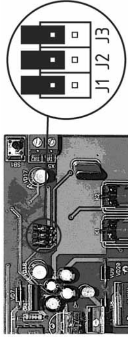
Рис 8. Положение перемычек прибора «Кварц» для программирования электронных ключей.
