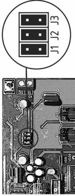
Рис 7. Положение перемычек прибора «Кварц» для программирования в режим охраны.
